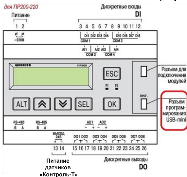
Рис. 1. Внешний вид и функциональные элементы контроллера
