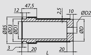
Рис. 2 Токоведущий стержень на ток до 2000 А
