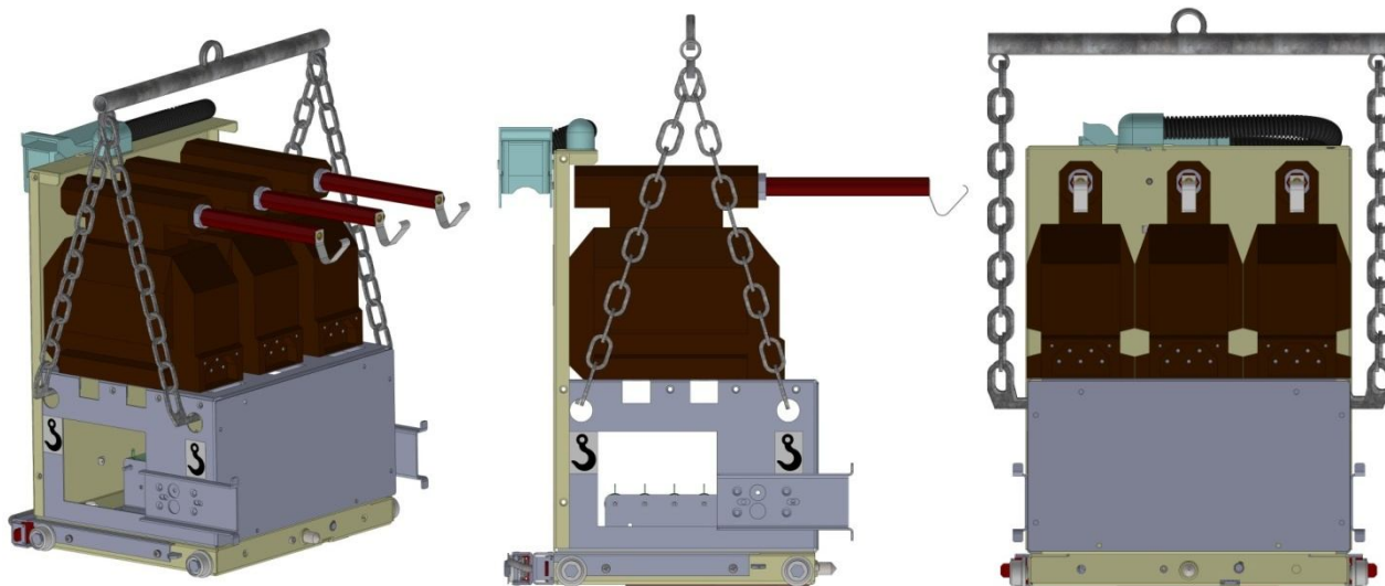
Рис. 18. Схема строповки выкатных элементов с трансформаторами напряжения
