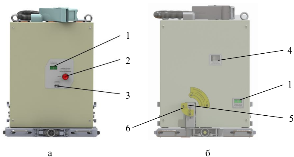
Рис. 3.1. Выкатной элемент с вакуумным выключателем: а - BB/TEL; б – SHELL; в – Evolis; г - Sion
