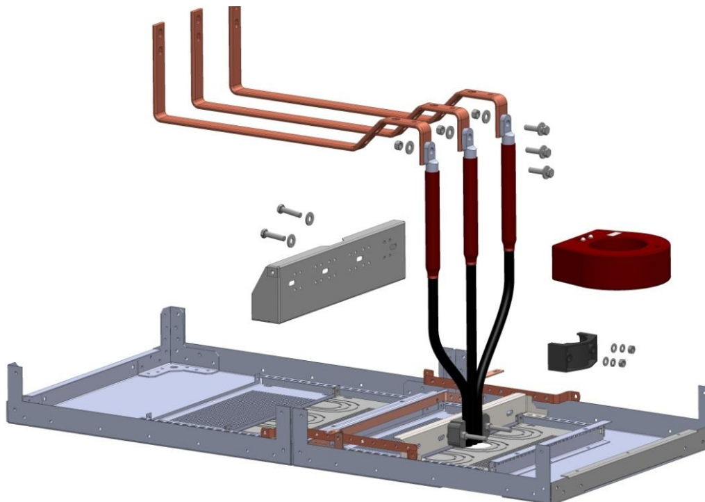
Рис. 31. Способ крепления элементов в отсеке кабельных присоединений
