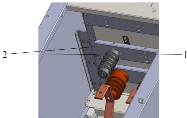
Рис. 38. Планка с ОПН
