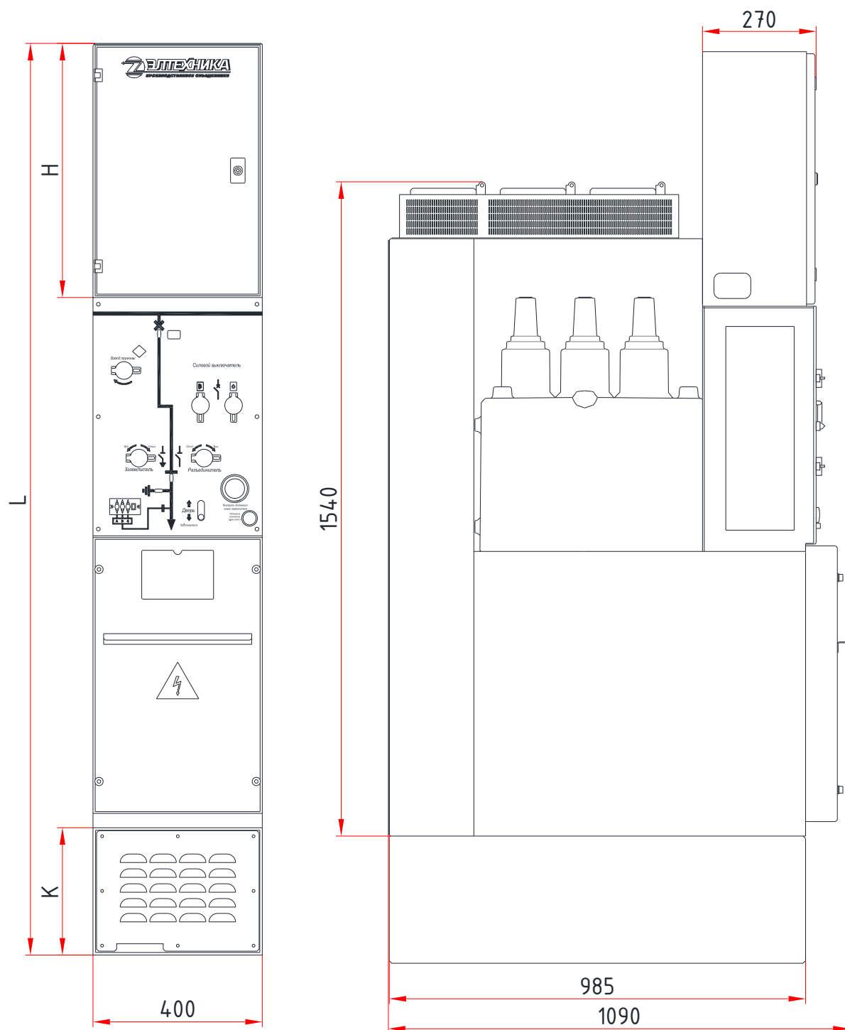
Рис. 2.5 Габаритные размеры шкафов КРУ на номинальный ток 1250А на цоколе Высота модуля вторичных цепей и цоколя определяется опционально, исходя из проектного задания. Размеры К, L и Н указаны в таблице, рис. 2.1.
