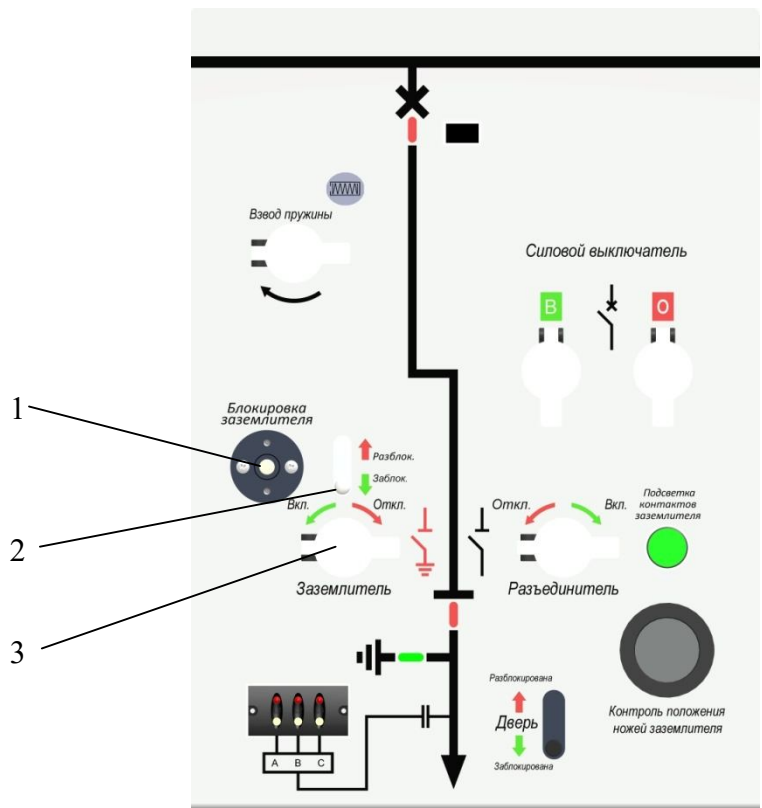
Рис. 8 Электромагнитная блокировка оперирования заземлителем
