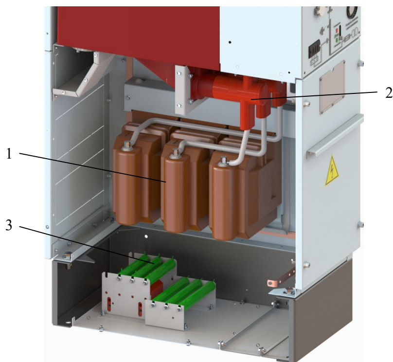
Рис. 11 Шкаф с измерительными трансформаторами напряжения на цоколе 200 мм 1 – трехфазная группа ТН типа ЗНОЛП; 2 – подключение ТН к бушингам; 3 – антиферрорезонансный комплект
