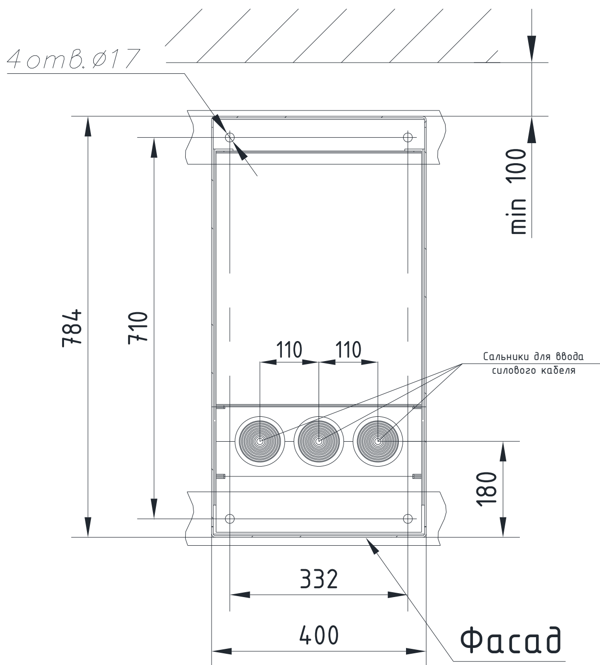
Рис. 3.1 Вид сверху на дно шкафа КРУ на номинальный ток 630А
