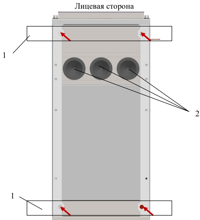
Рис. 14 Размещение закладных швеллеров и отверстий для прохода силовых и контрольных кабелей. 1 – швеллер №10 – 2 шт.; 2 – сальники для ввода силового кабеля диаметром до 90 мм
