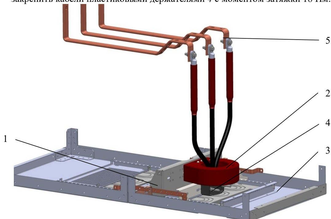
Рис. 30. Монтаж кабеля в отсеке кабельных соединений
