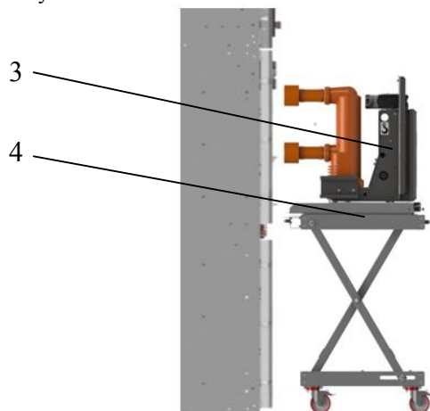
Рис. 18. Порядок демонтажа выкатного элемента
