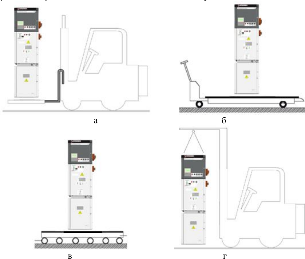
Рис. 16. Способы перемещения шкафов КРУ на транспортном поддоне
