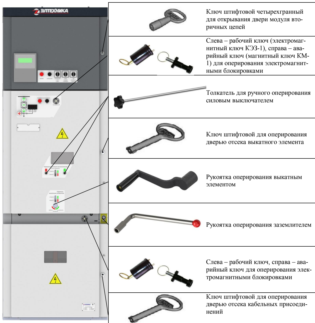
Рис. 3. Принадлежности КРУ
