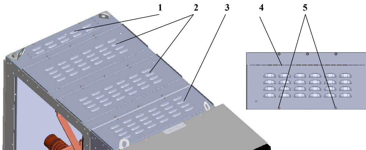
Рис. 13. Клапаны сброса давления:
