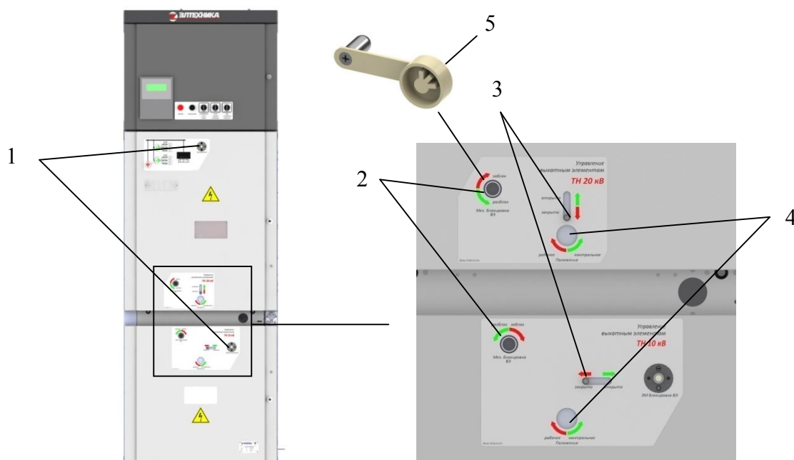
Рис. 10.1 Шкаф с измерительными трансформаторами напряжения
