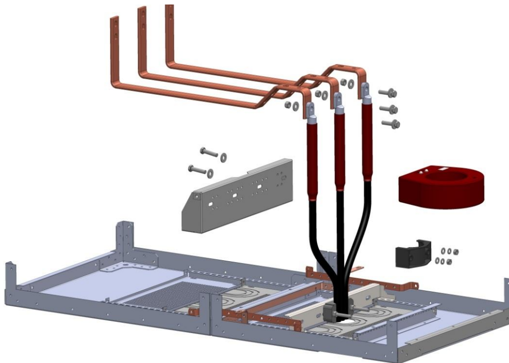
Рис. 30 Способ крепления элементов в отсеке кабельных присоединений
