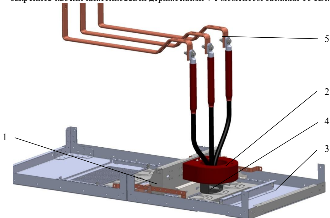
Рис. 29 Монтаж кабеля в отсеке кабельных присоединений
