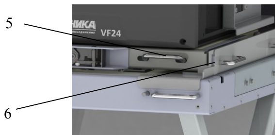
Рис. 18. Порядок демонтажа выкатного элемента
