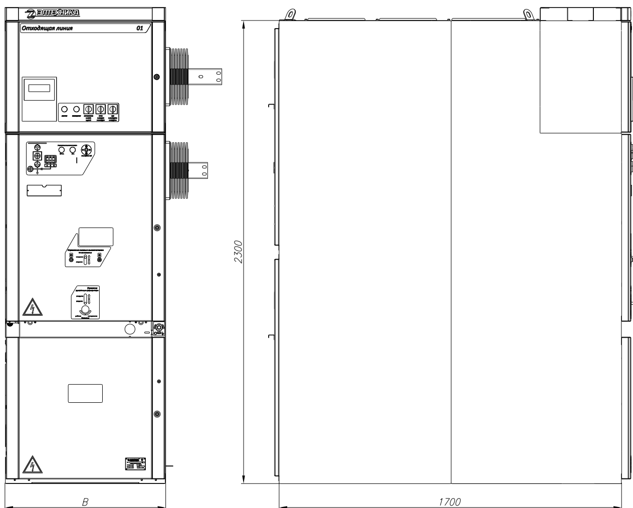
Рис. 2.1. Габаритные размеры шкафов КРУ
