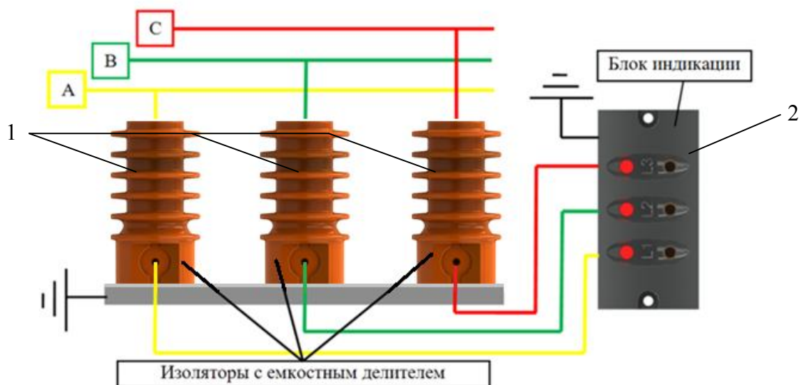
Рис. 11. Схема соединения блока индикации напряжения
