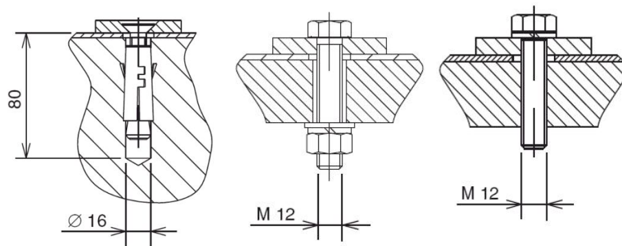
Рис. 20. Способы крепления шкафов КРУ
