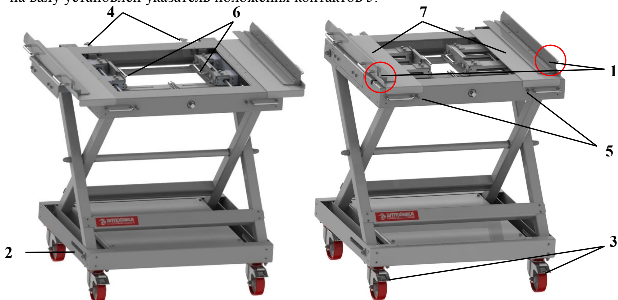
Рис. 9. Сервисная тележка:
