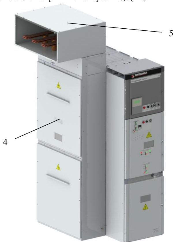
Рис. 36. Сборка шинного ввода сбоку шкафа КРУ
