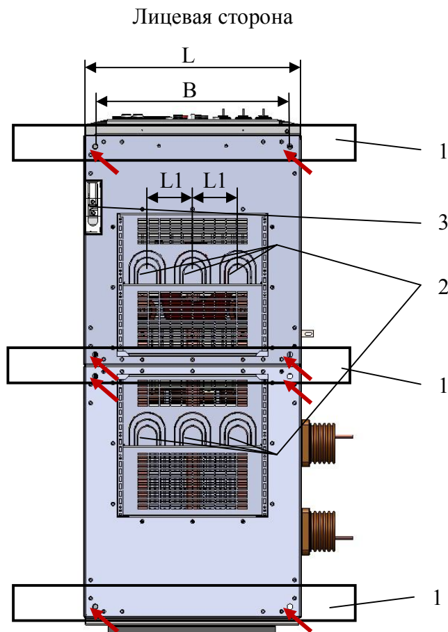
Рис. 19. Установочные размеры шкафов КРУ, размещение закладных швеллеров и отверстий для прохода силовых и контрольных кабелей. Вид сверху на дно шкафа КРУ
