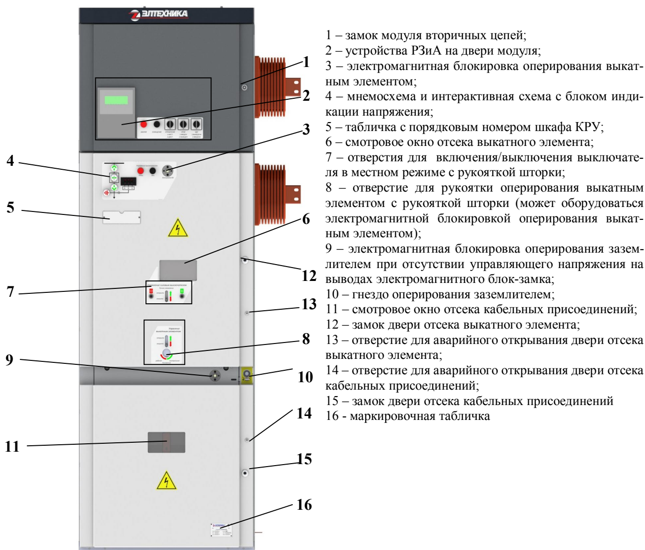
Рис. 2. Лицевая сторона КРУ
