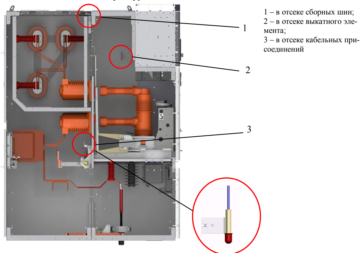
Рис. 14. Места установки датчиков дуговой защиты в отсеках шкафа КРУ
