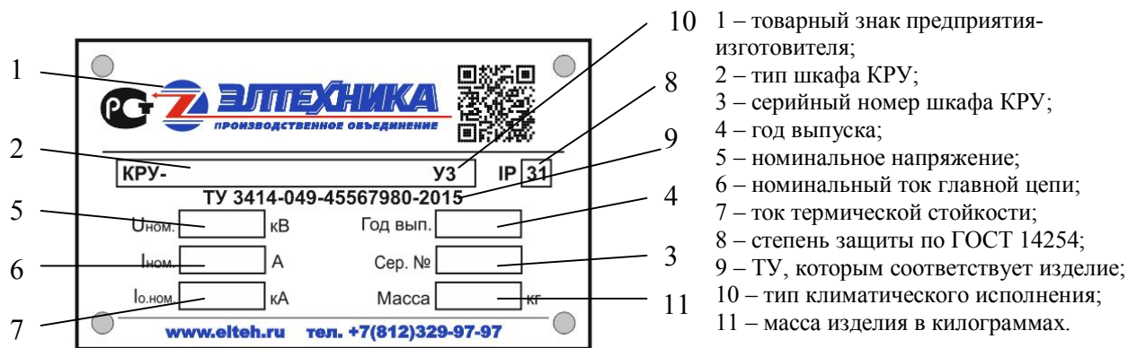
Рис. 5. Маркировочная табличка
