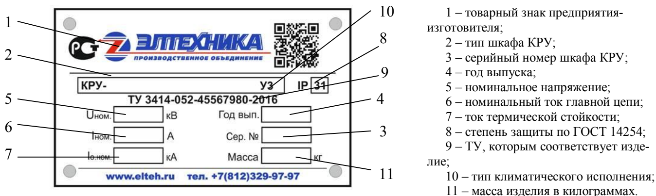
Рис. 5 Маркировочная табличка
