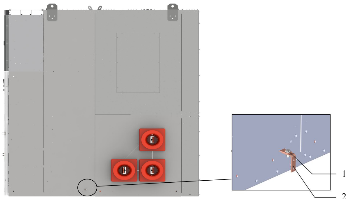
Рис. 20 Сборка системы заземления секции КРУ
