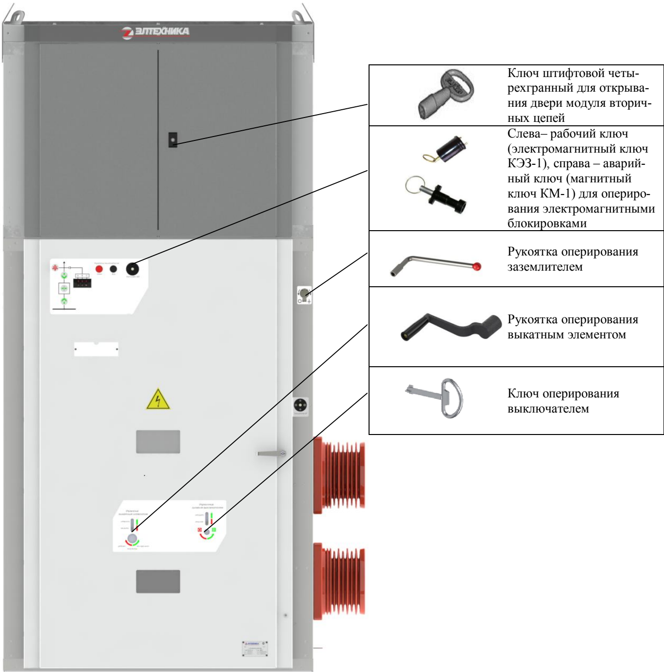
Рис. 3 Принадлежности КРУ
