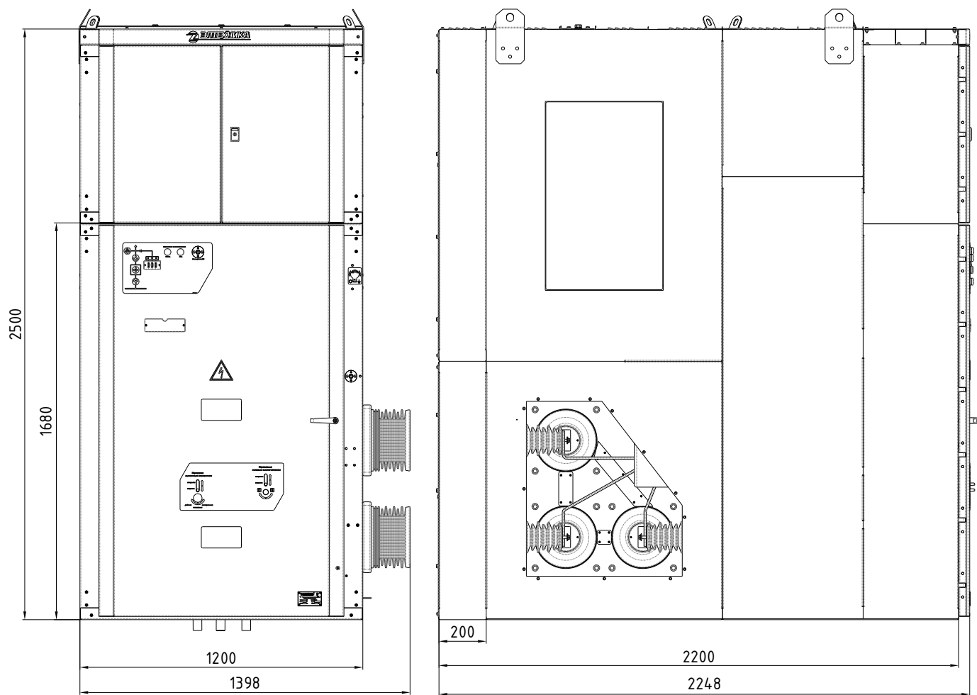
Рис. 2.1 Габаритные размеры шкафов КРУ с нижним расположением сборных шин
