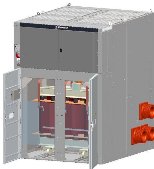
Рис. 23 Монтаж трансформатора собственных нужд
