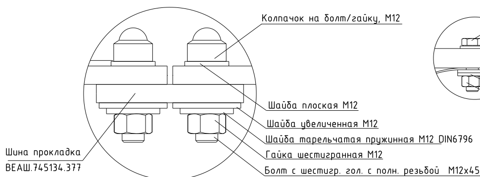
Рис. 22 Монтаж сборных шин 1600 А (вид снизу на шкафы КРУ)
