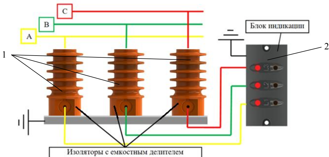
Рис. 12 Схема соединения блока индикации напряжения
