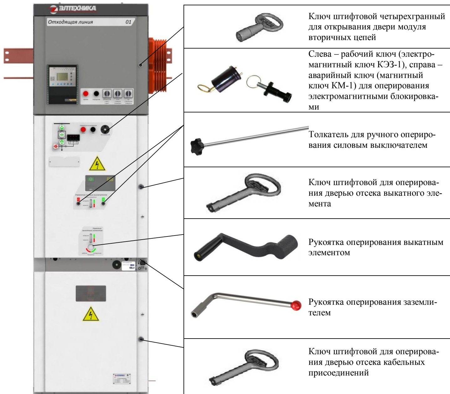
Рис. 3 Принадлежности шкафа КРУ
