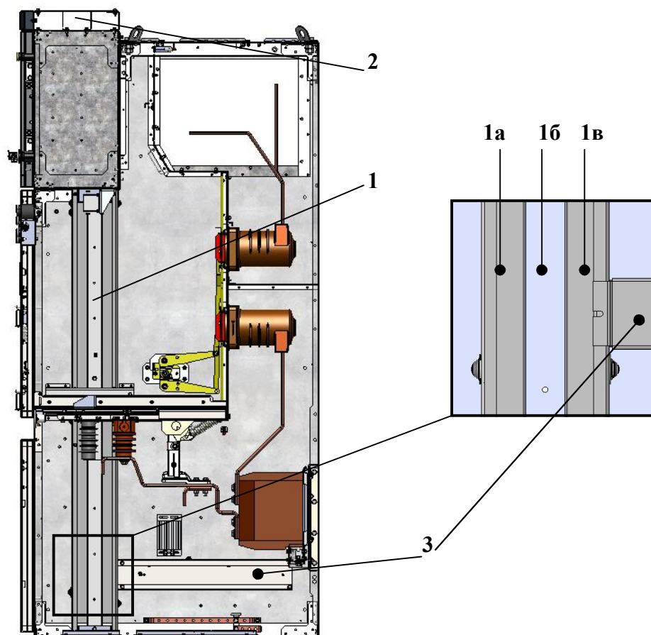
Рис. 15А. Кабельные каналы для прокладки жгутов проводников вторичных цепей
