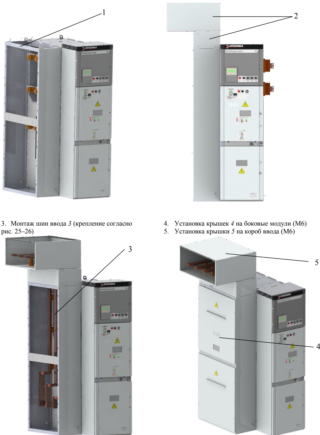
Рис. 31. Сборка шинного ввода сбоку шкафа КРУ
