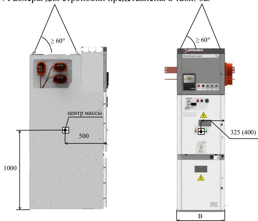
Рис. 17 Схема строповки шкафов КРУ
