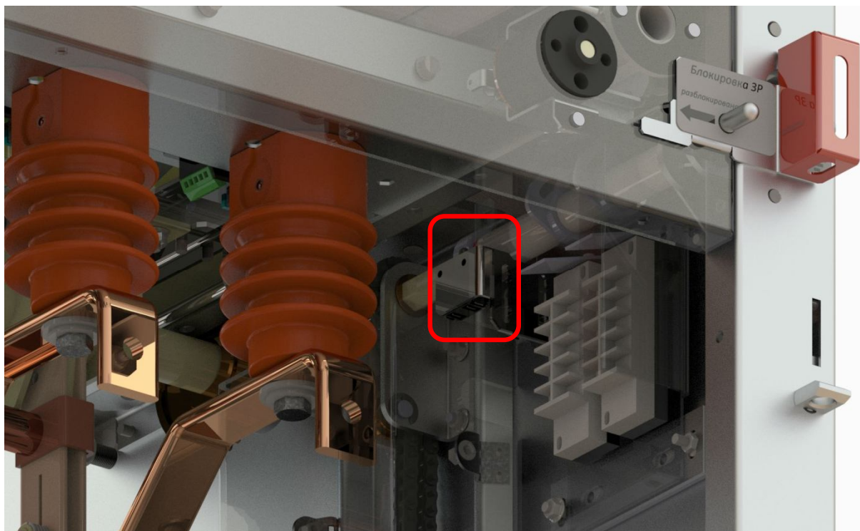
Рис. 5.1 Внешний вид концевых переключателей моторизованного привода заземлителя.
