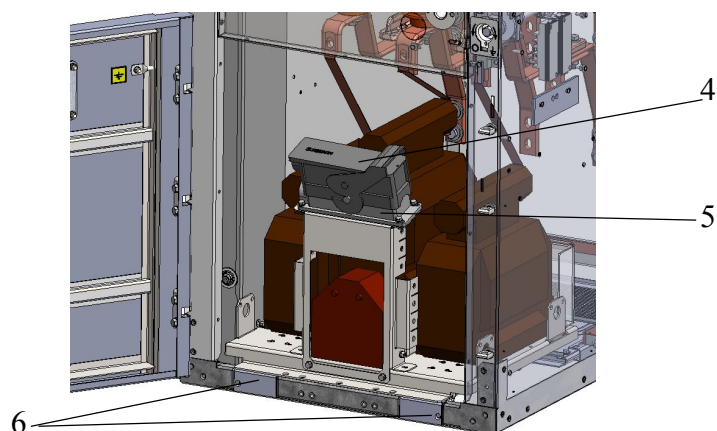
Рис. 286. Порядок монтажа выкатного элемента с измерительными трансформаторами напряжения в отсек кабельных присоединений
