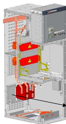
Рис. 34 Порядок демонтажа измерительных трансформаторов тока
