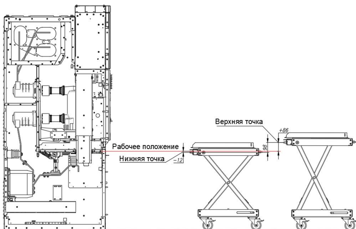
Рис. 10а Диапазон регулировки сервисной тележки по высоте
