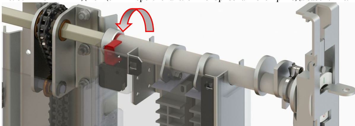
Рис. 5.2 Крайнее положение привода вала (заземлитель в положении «Отключен»).
