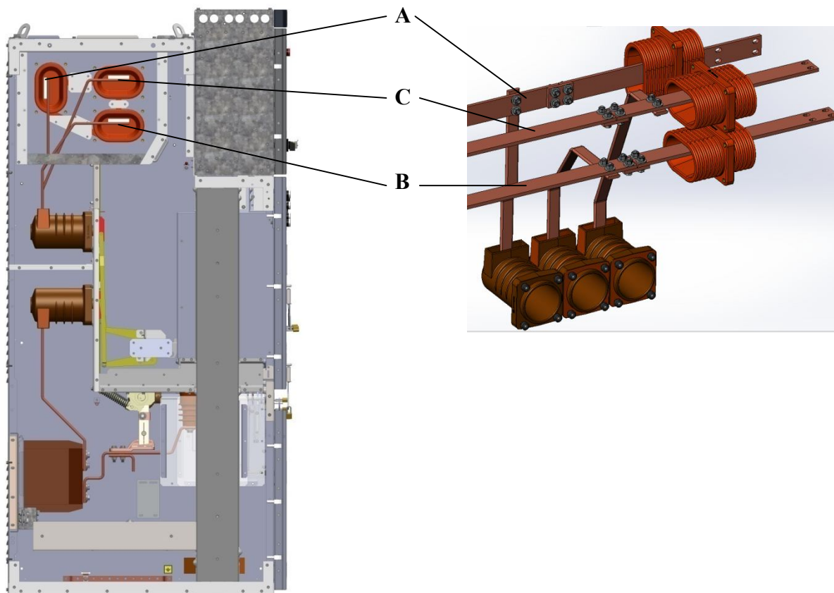
Рис. 25. Монтаж сборных шин
