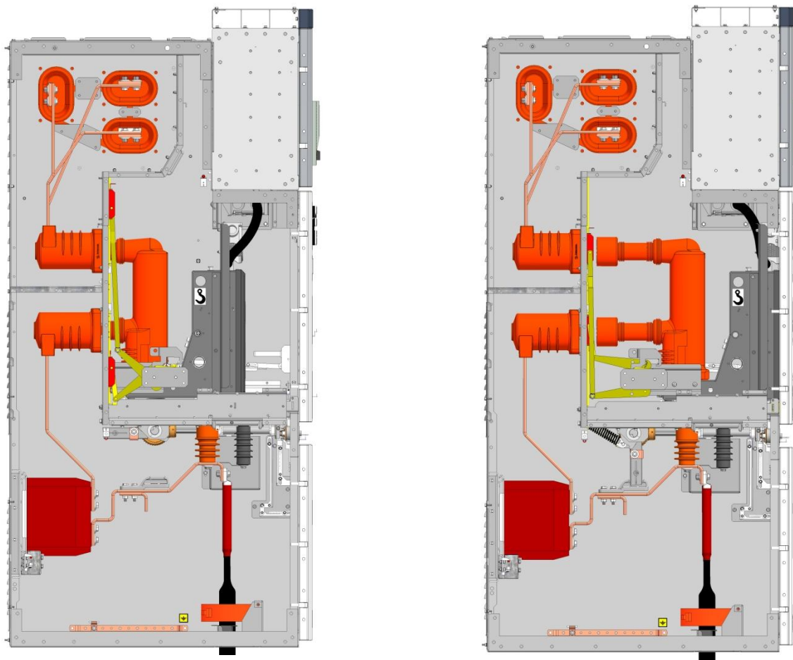
Рис. 7 Положения выкатных элементов на примере силового выключателя VF12 (слева – рабочее, справа – контрольное)
