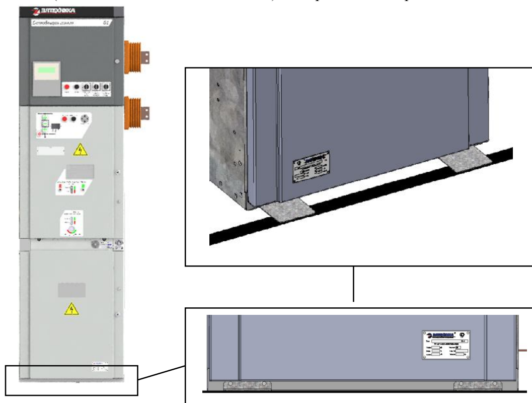
Рис. 24 Присоединение к внешнему контуру заземления
