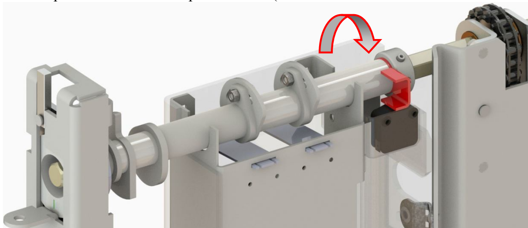
Рис. 5.3 Крайнее положение привода вала (заземлитель в положении «Заземлен»).
