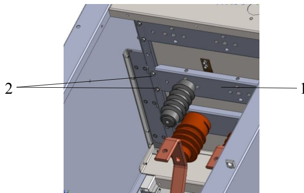
Рис. 33 Планка с ОПН
