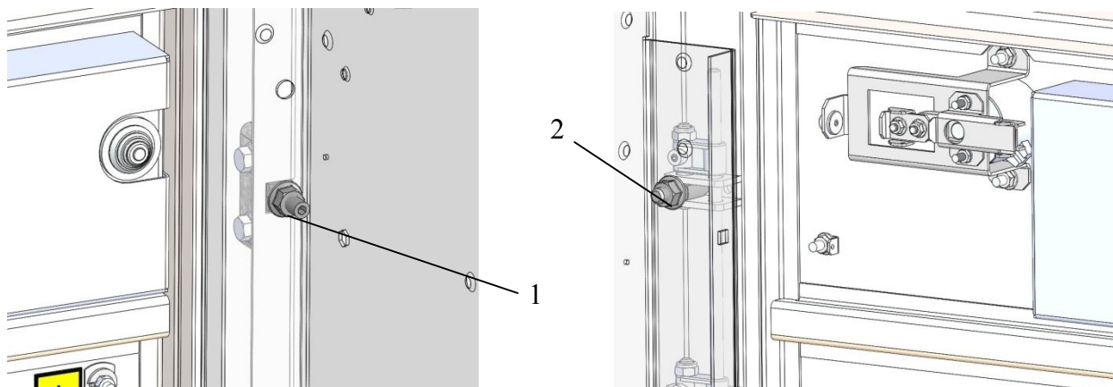
Рис. 32 Крепление петель дверей и проушин замка (вид изнутри)
