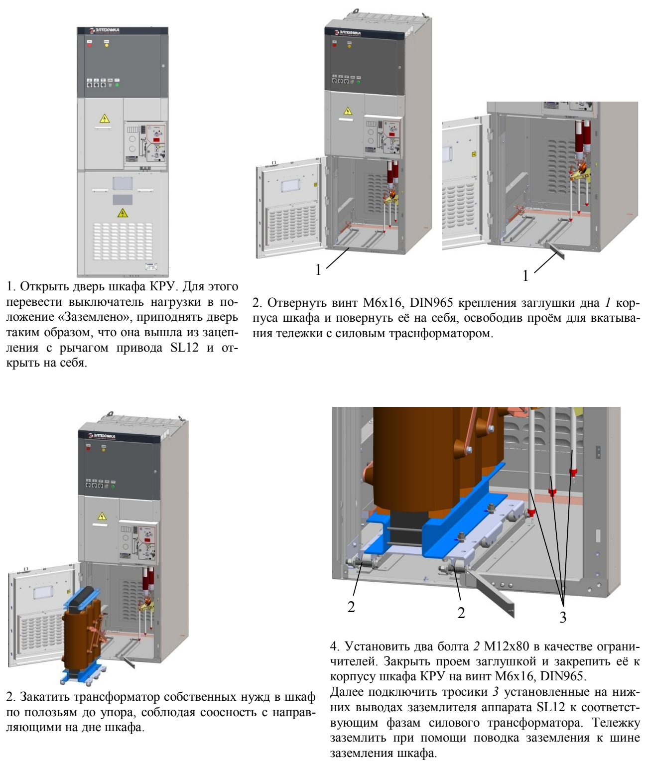
Рис. 6.3 Порядок монтажа выкатного элемента с трансформатором собственных нужд в шкаф
