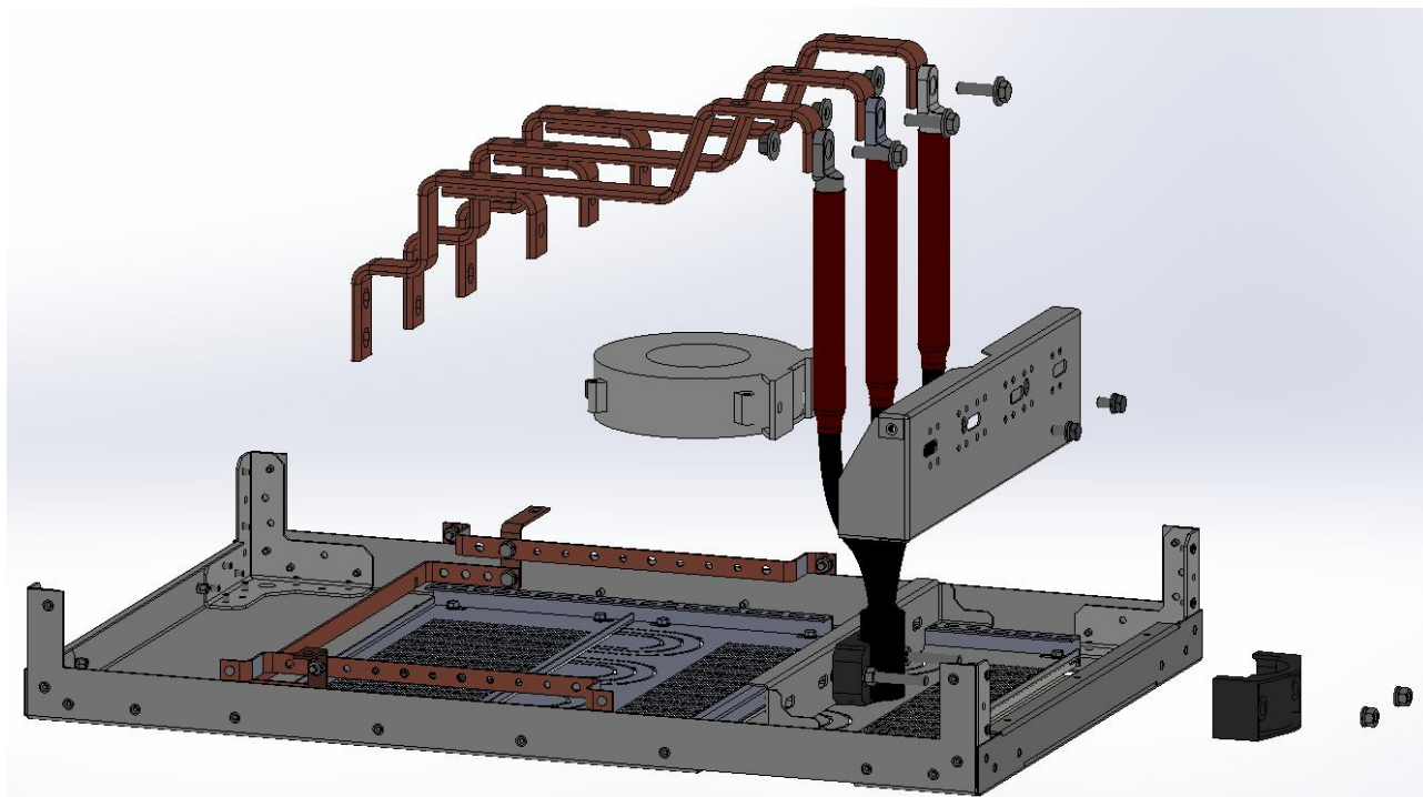
Рис. 28. Способ крепления элементов в отсеке кабельных присоединений
