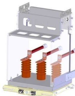
выводы для испытания кабелей повышенным напряжением
