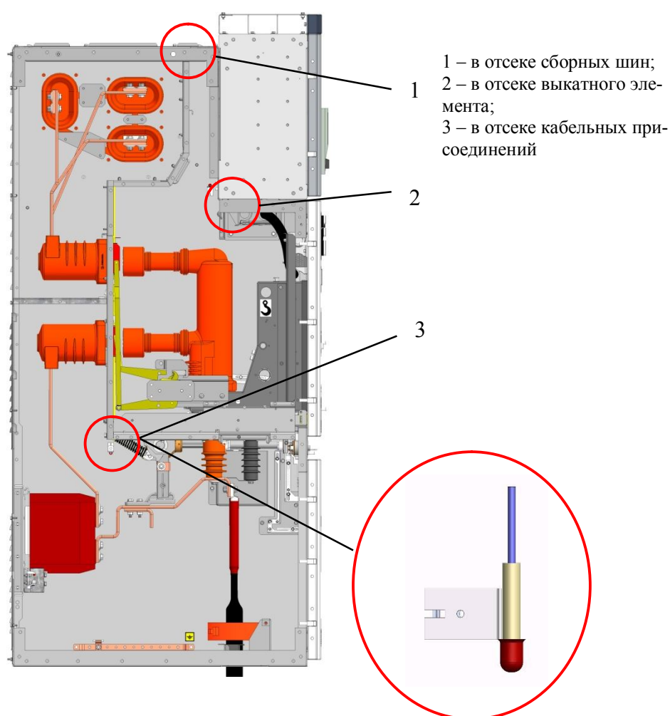
Рис. 15 Места установки датчиков дуговой защиты в отсеках шкафа КРУ
