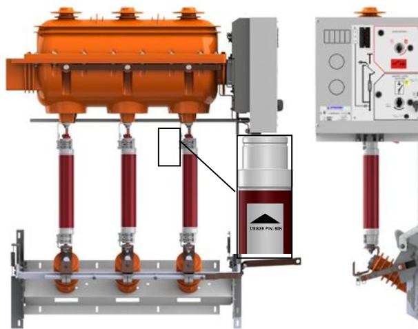
Рис. 6.4 Предохранители
