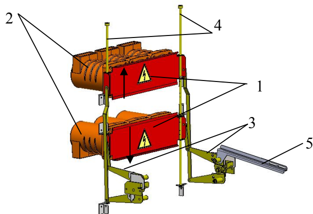
Рис. 11 Шторочный механизм
