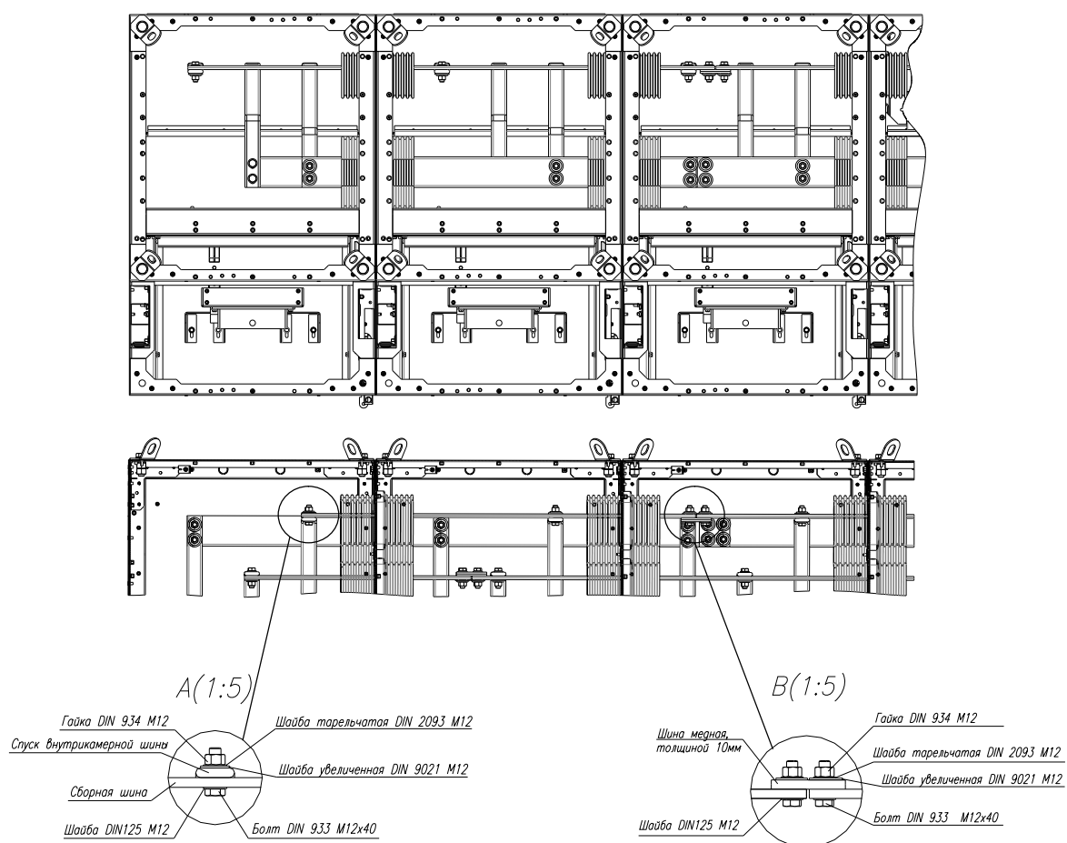
Рис. 26 Монтаж сборных шин (вид сверху на шкафы КРУ)
