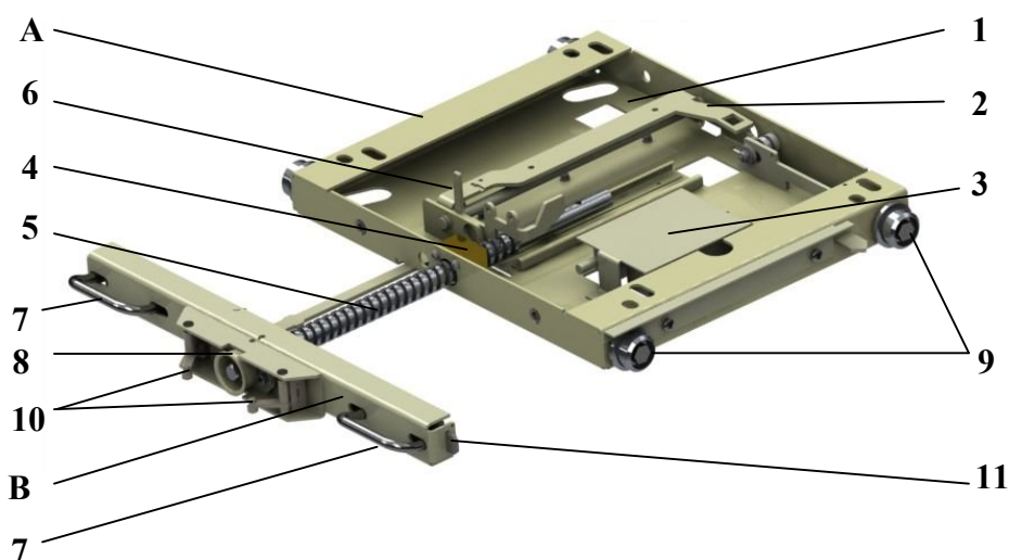
Рис. 8 Тележка аппаратная:
