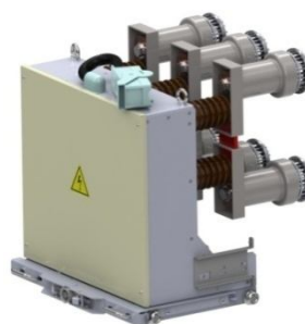
секционный разъединитель
