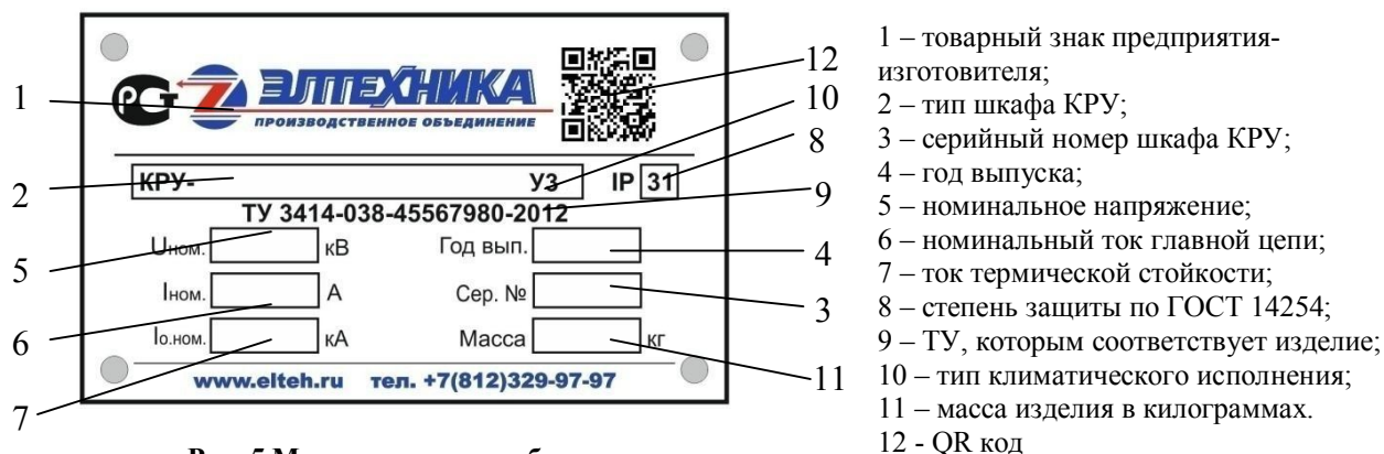
Рис. 5 Маркировочная табличка
