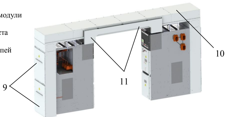
Рис. 29. Сборка шинного моста
