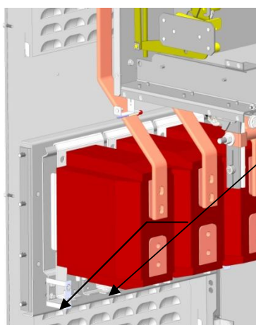
Рис. 34 Порядок демонтажа измерительных трансформаторов тока
