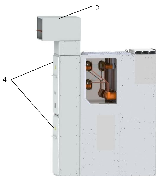
Рис. 30. Сборка шинного ввода сзади шкафа КРУ
