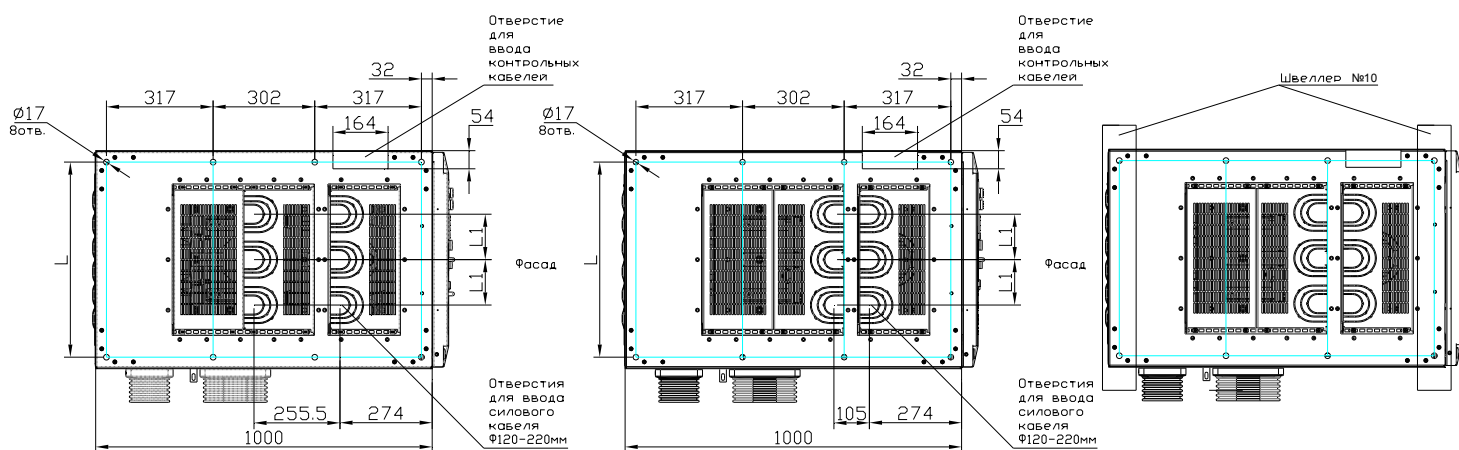
Рис. 2.2 Установочные размеры шкафов КРУ (вид снизу)
