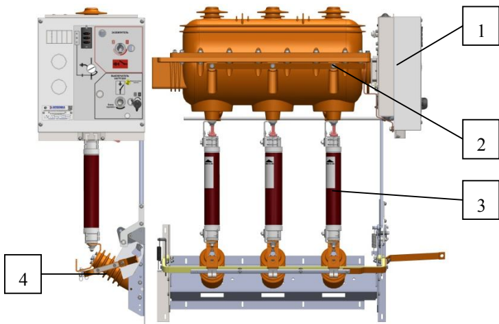
Рис. 6. Общий вид аппаратов на примере SL12(24)-BH(A, B):
