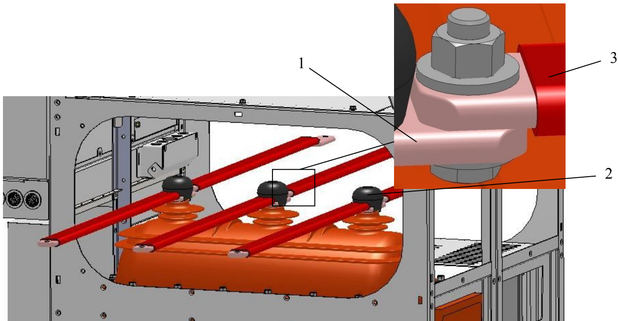
Рис. 4.3 Общий вид отсека сборных шин КСО 20 кВ
