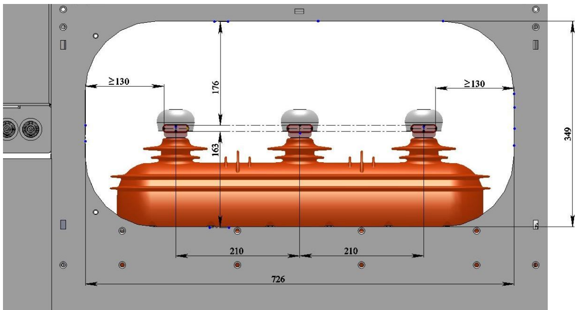
Рис. 4.4 Минимально допустимые расстояния от токоведущих шин до заземленных частей корпуса КСО 20 кВ
