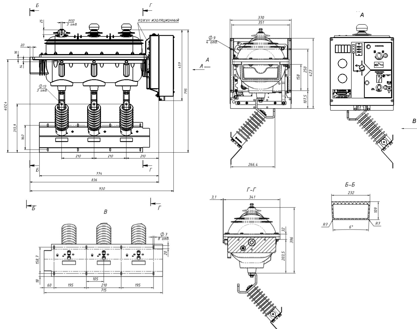
Рис. 1.11 Габаритно-присоединительные размеры аппарата типов SL24-BH(I, J), SL24-BT(I, J), SL24-DH(I, J)
