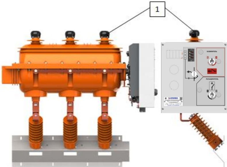
Рис. 14а. Общий вид аппаратов SL24B(Д):
