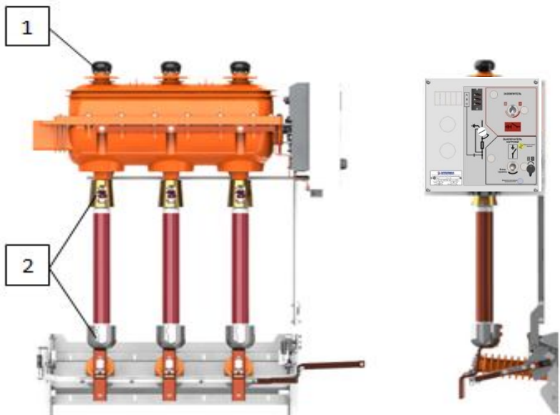
Рис. 14б. Общий вид аппаратов SL24BTA(В):
